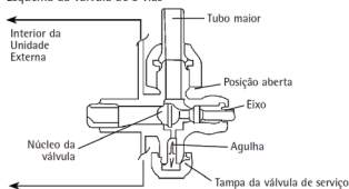
Esquema da válvula de 3 vias
