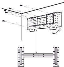
PERFURAÇÃO DA PAREDE PARA PASSAGEM DOS TUBOS.
