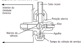
Esquema da válvula de 3 vias
