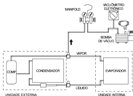
Válvulas da Unidade Externa
