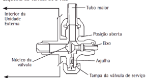
Esquema da válvula de 3 vias
